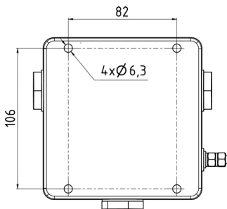
Установочные размеры
